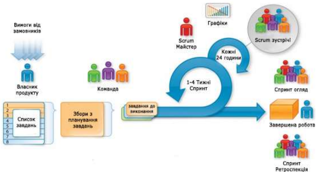
Рис. 4. Опис Scrum-процесу
