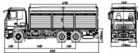
Схема зернобоза МАЗ-6501С9-8525-000
