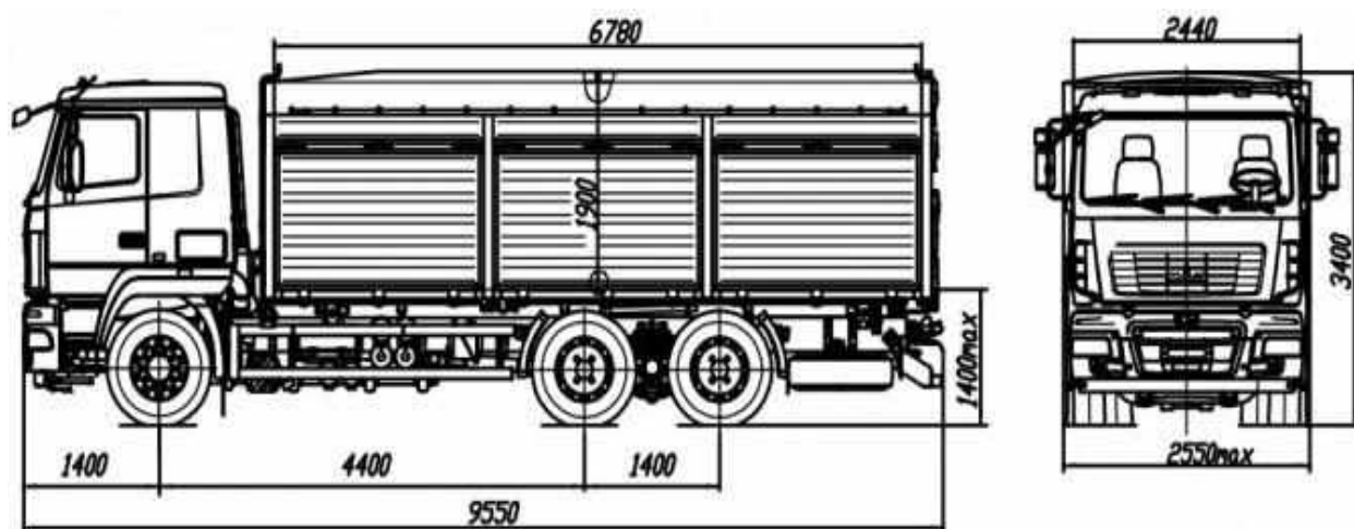
Рисунок 2.5 – Схема зерновоза МАЗ-6501С9-8525-000 (розроблено за [20])
